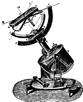
FIG. 3—Silbermann's Heliostat.
