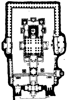
FIG. 5.—Plan of Kailās at Ellora.
